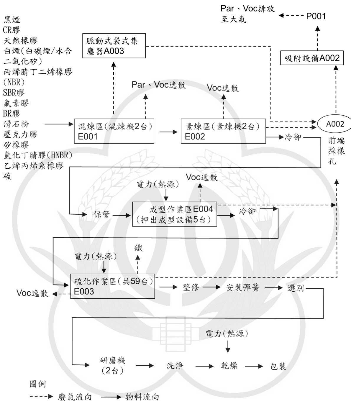
圖 1 其他橡膠製品製造程序製程流程圖
